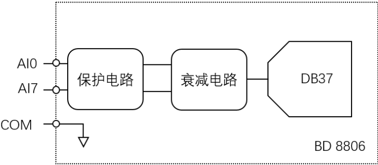
BD 8806 某通道的电路示意图
